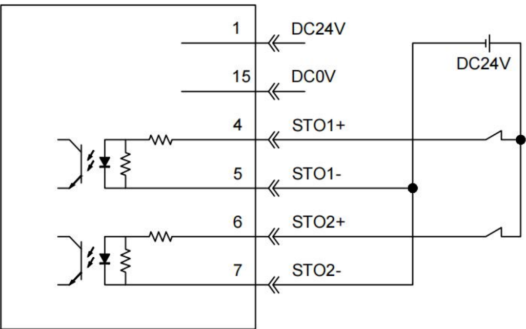
ST0接外部24V电源
