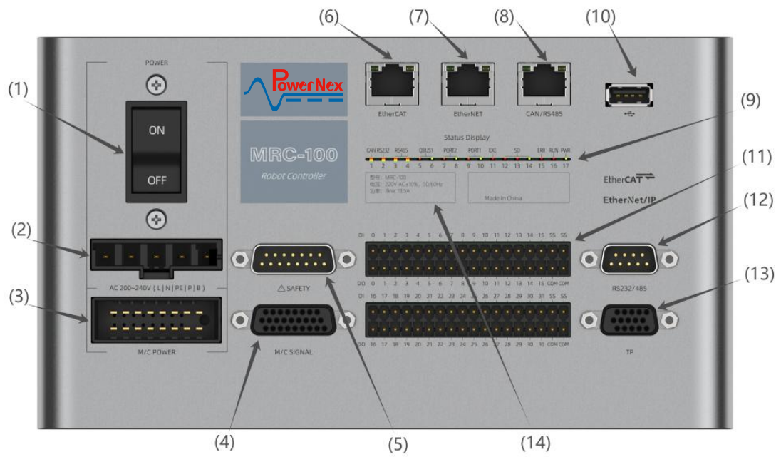
图 1-1 部件信息
