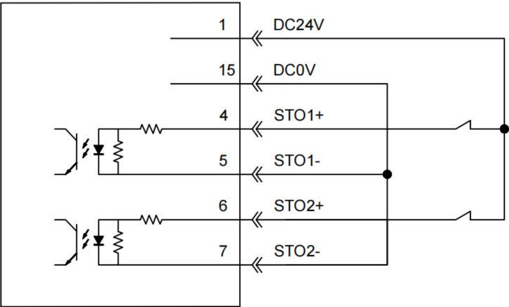
ST0接内部24V电源
