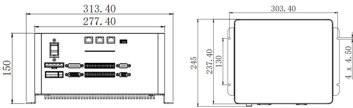
设备尺寸：长：277.40MM 宽：237.40MM 高：150MM 适用于 S 系列 【单位：mm】
