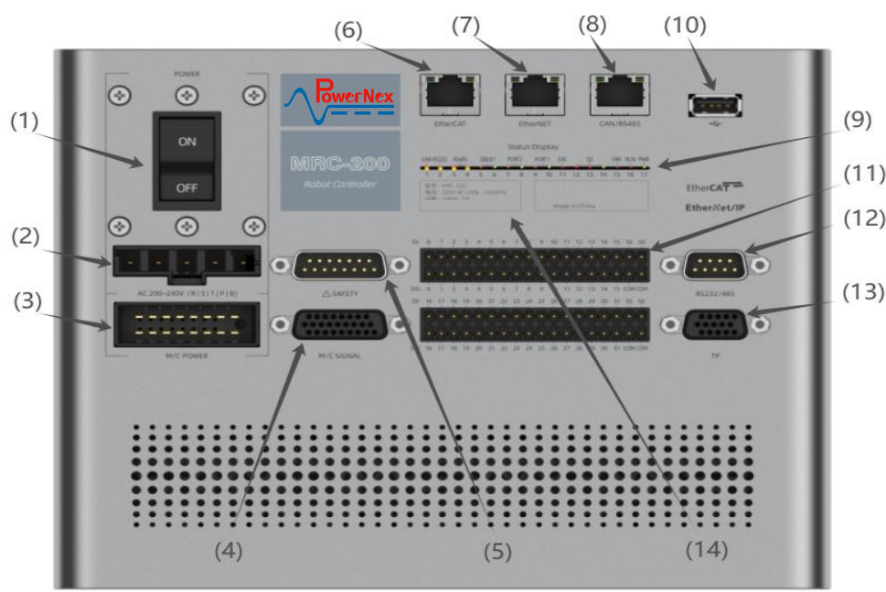
图 1-2 部件信息
