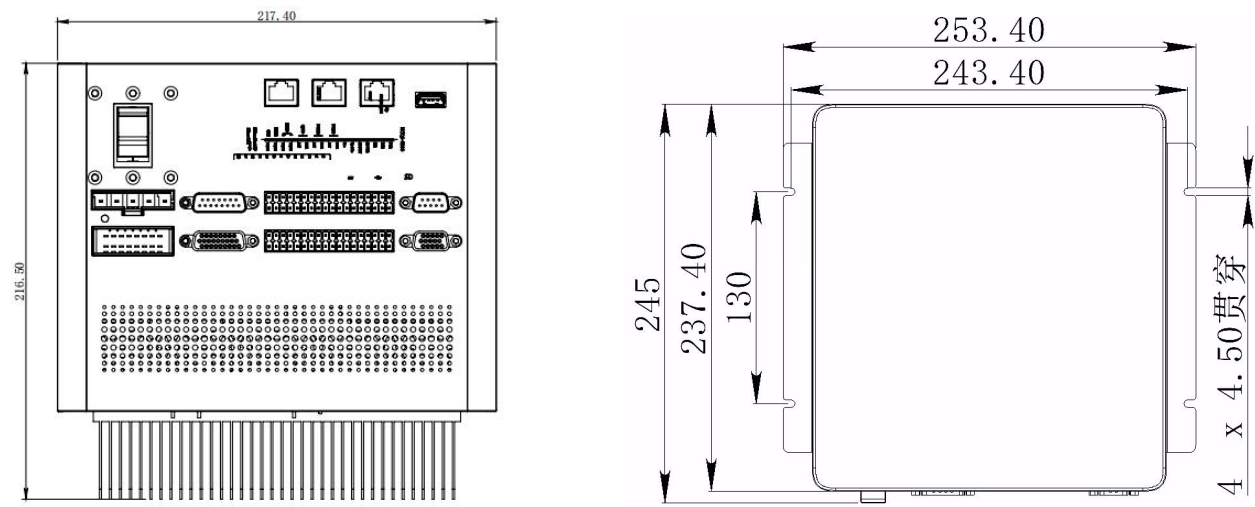
设备尺寸：长：217.40MM 宽：237.40MM 高：216.50MM 适用于 P60-P100 系列 【单位：mm】
